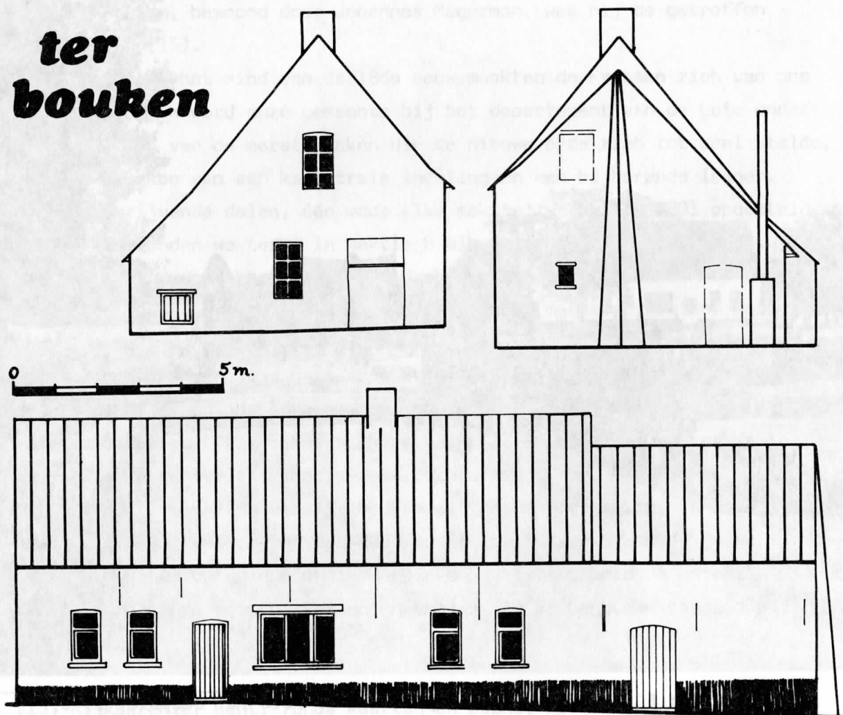
Fig 7 : Opmeting woonhuis
