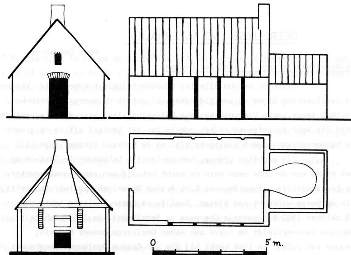
Fig 8 : Opmeting bakhuis
